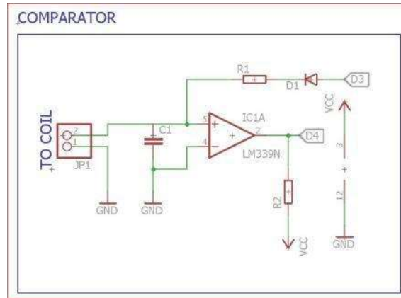
Gambar 3. Rangkaian Sensor Logam
